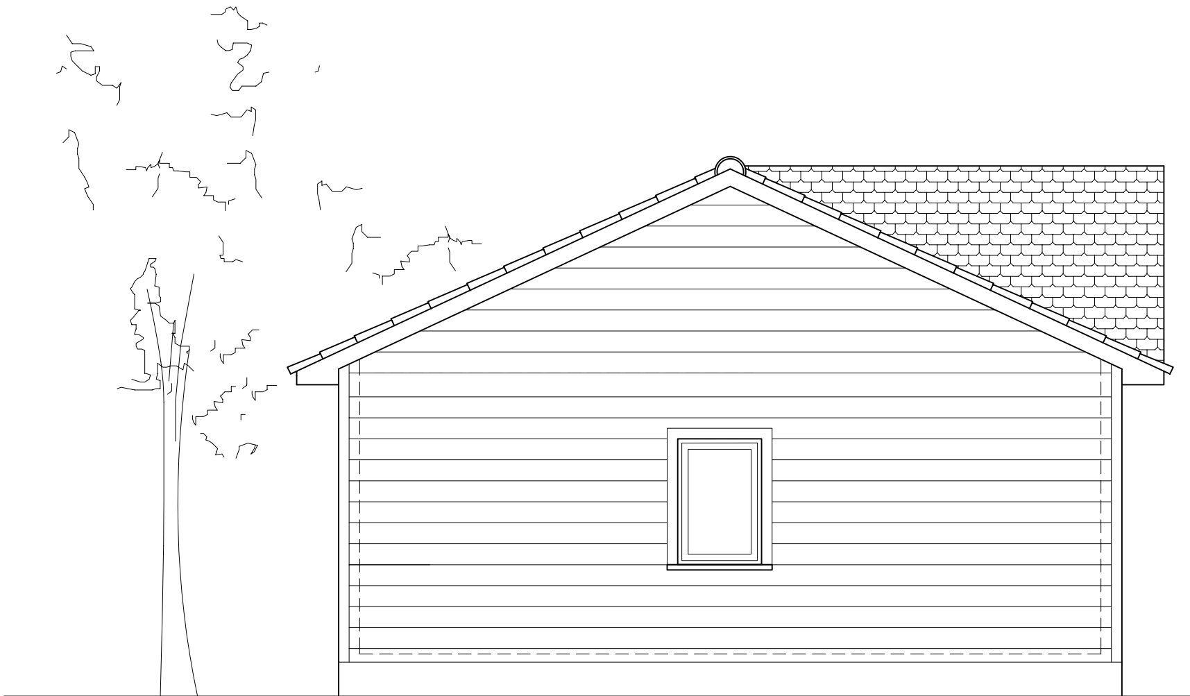
ALZADO LATERAL IZQUIERDO
